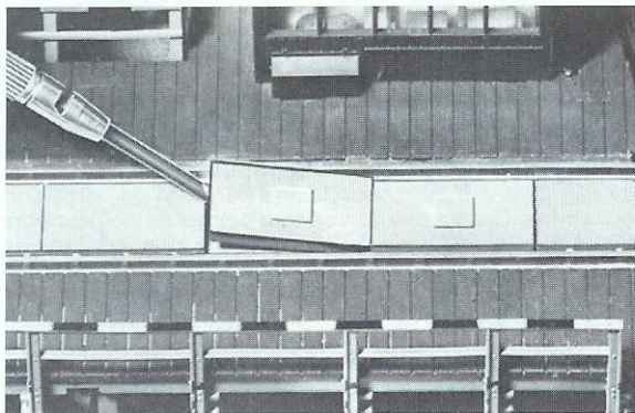
Fig. 13 Um die Lager des Antriebsmotors ölen zu können, muss die Gitterabdeckung vor dem Maschinenhaus mit einem kleinen Schraubendreher abgehoben werden.
