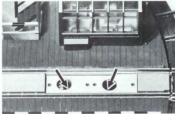
Fig. 14 Durch die vorgesehenen Löcher ist je 1 Tropfen Öl an die durch Pfeile gekennzeichneten Lagerstellen zu geben. Vorsicht, nicht überölen! Nur FLEISCHMANN-Öl 6599 verwenden. Zur Dosierung die in der Verschlusskappe der Ölflasche angebrachte Nadel verwenden.
